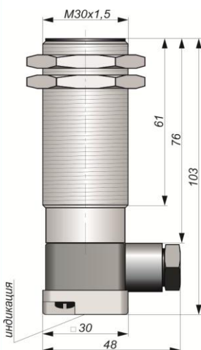
Габаритный чертеж
