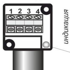
Цоколевка клеммной колодки
